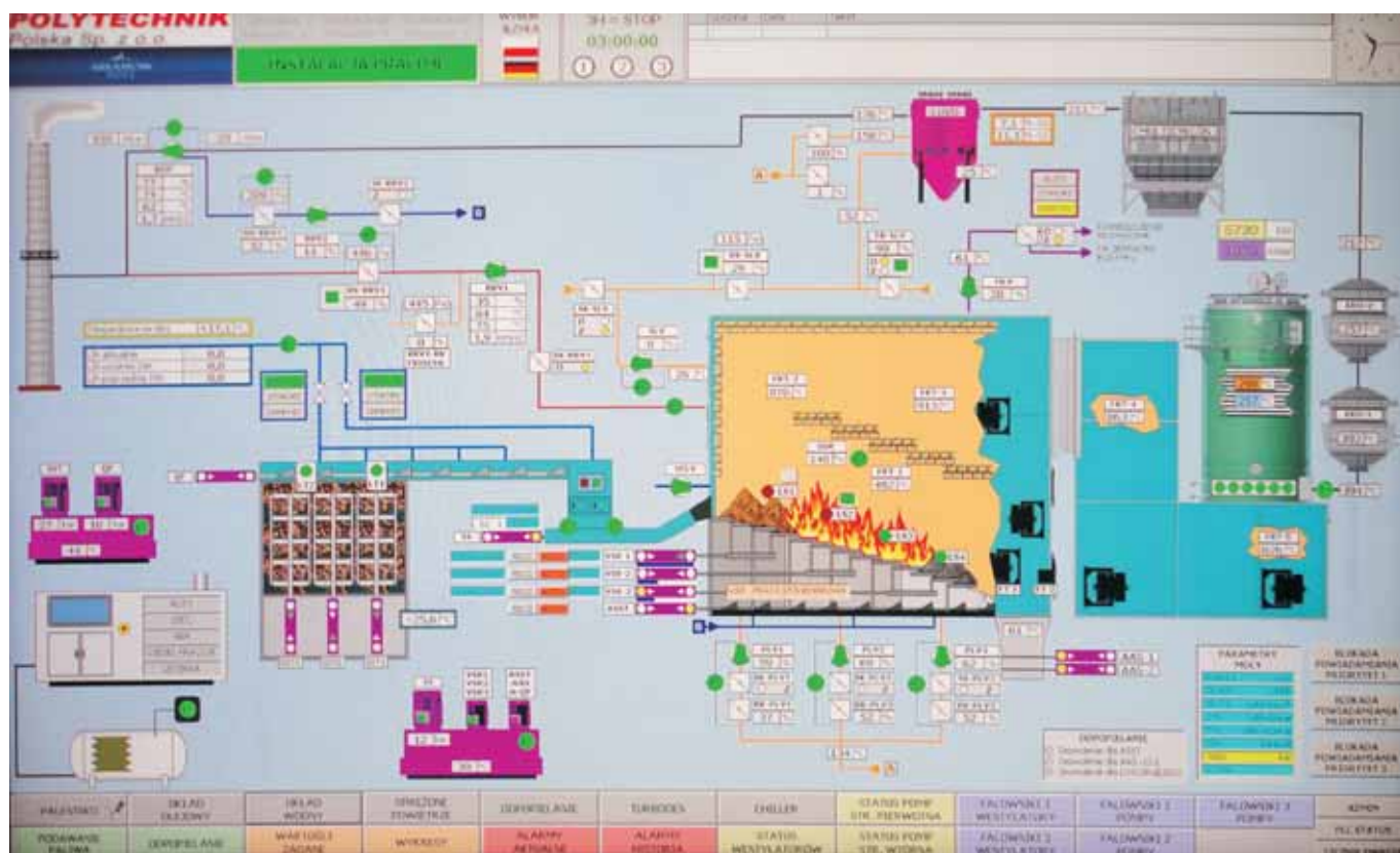
Wizualizacja układu technologicznego.
